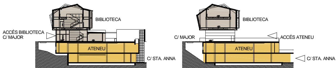
SECCIONS TRANSVERSALS
