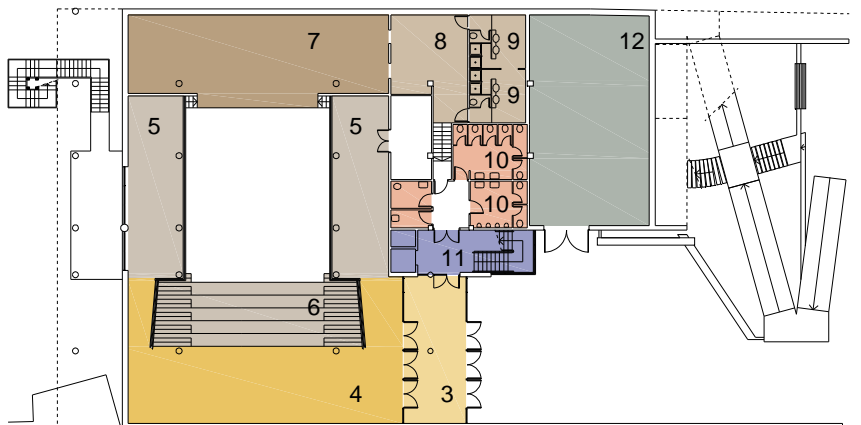
PLANTA BAIXA
