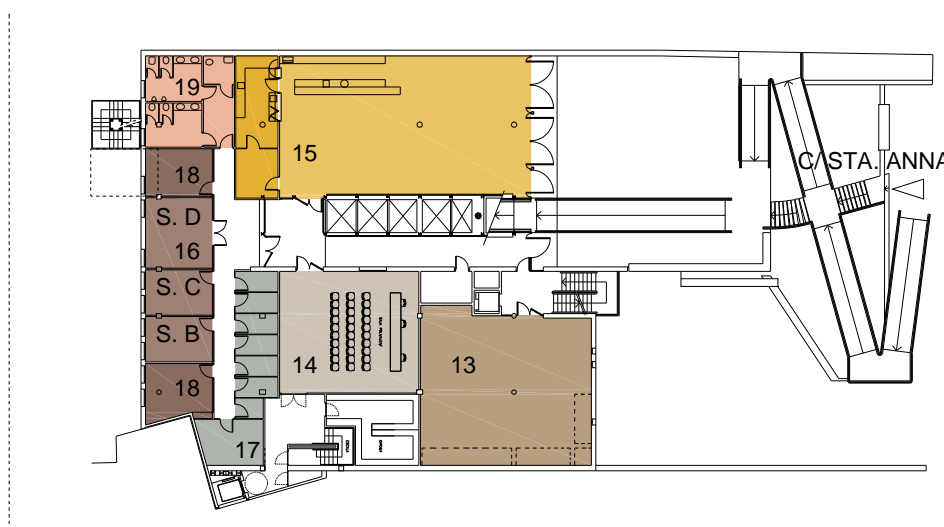
PLANTA PRIMERA
